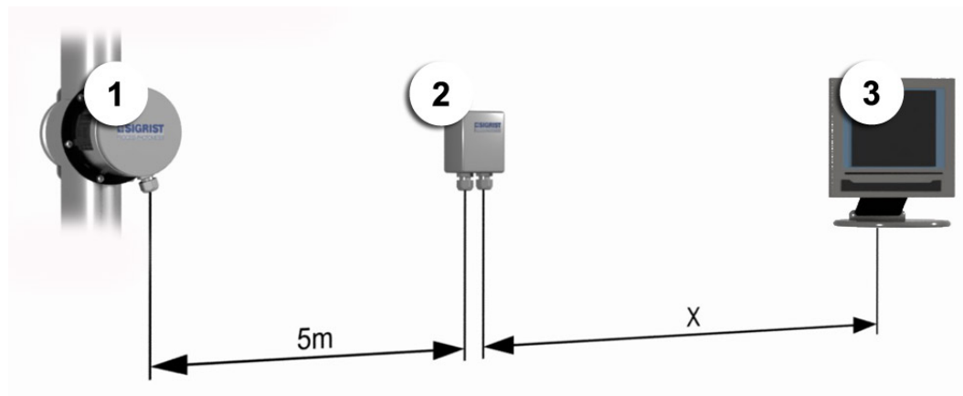
Abbildung 6: Installation des Photometers mit Anschlussdose
