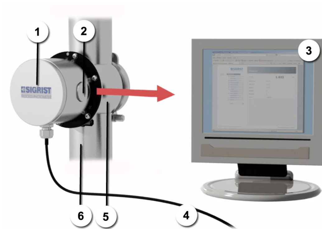
Abbildung 1: Gesamtansicht TurbiGuard
