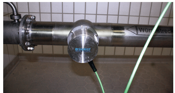
PhaseGuard C in Würzeleitung
